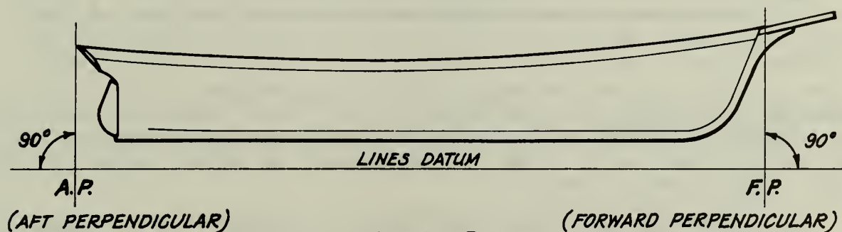
Fig. 4.2.7 Perpendiculars
